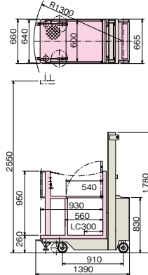
■外形寸法図
