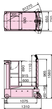
■外形寸法図
