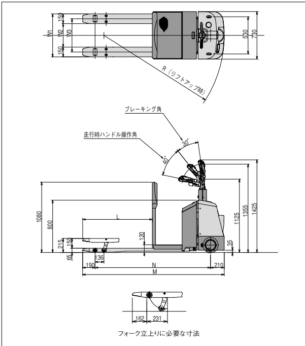
二面図
